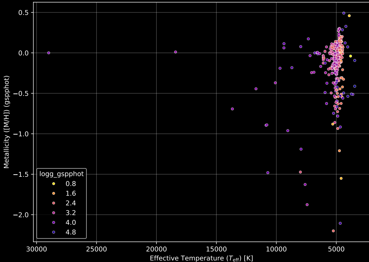
APOGEE DR17 Field: [090-04] Stellar Population Parameters (n= 406)
